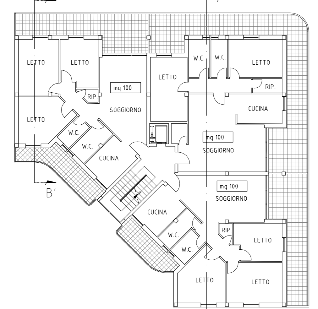
PIANTA PIANO TIPO
