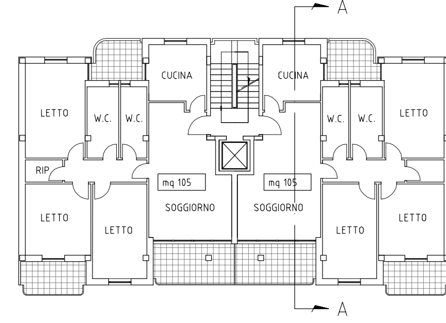
PIANTA PIANO II, III e IV
