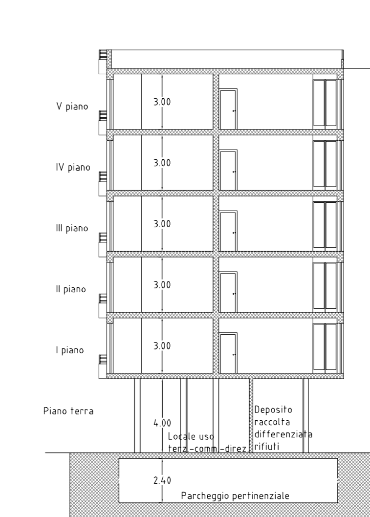
SEZIONE D-D
