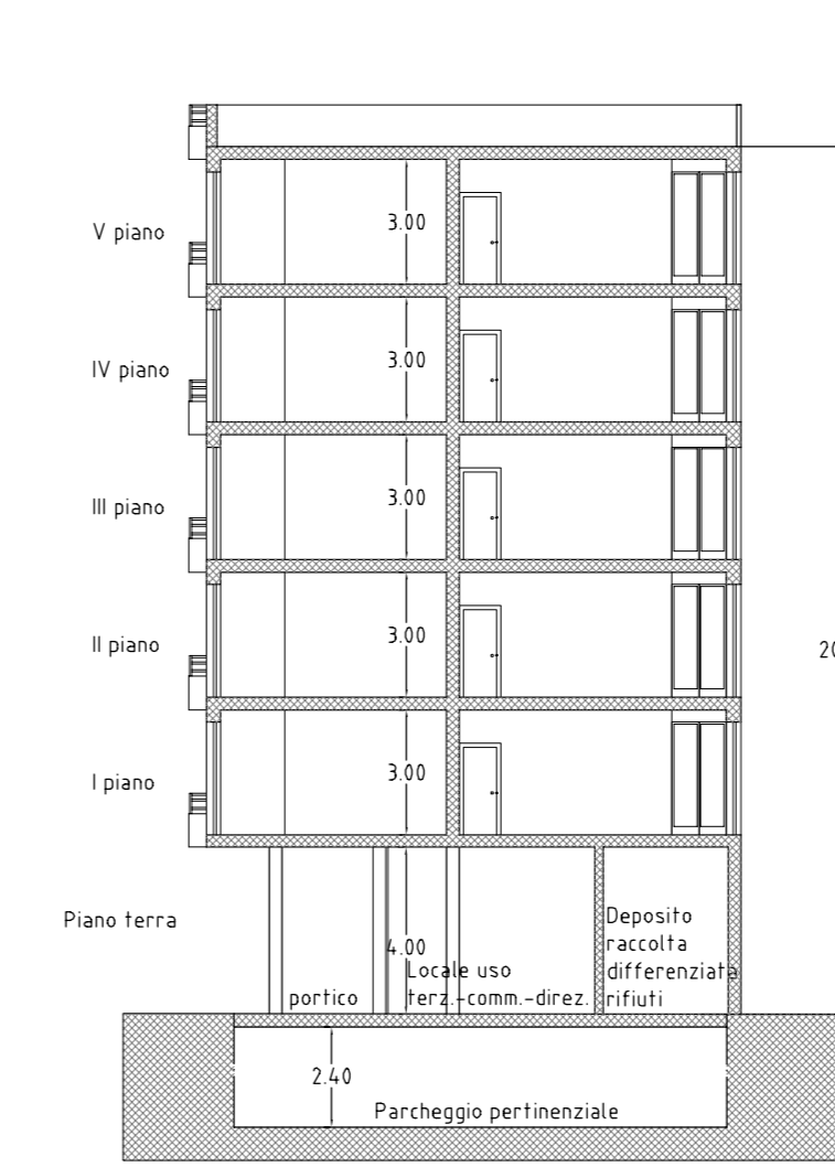
SEZIONE C-C
