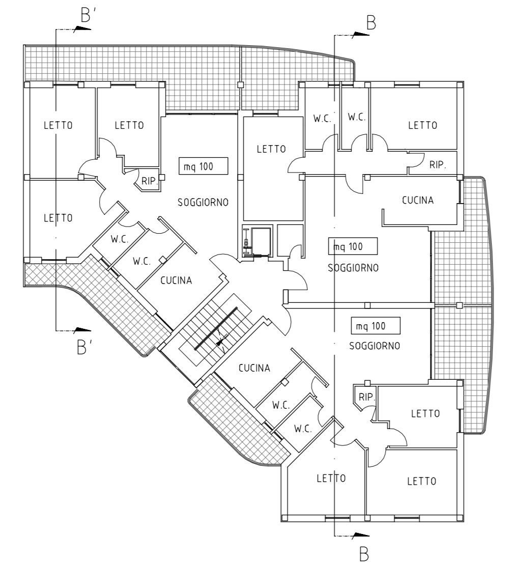
PIANTA COPERTURA
