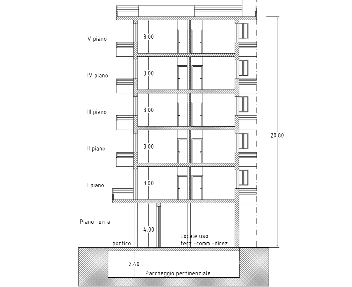
SEZIONE B1-B1
