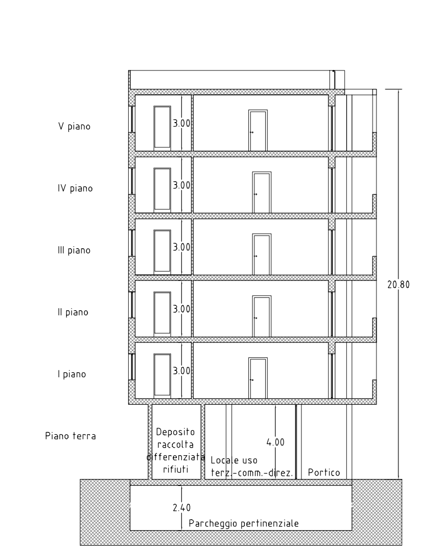
SEZIONE A-A
