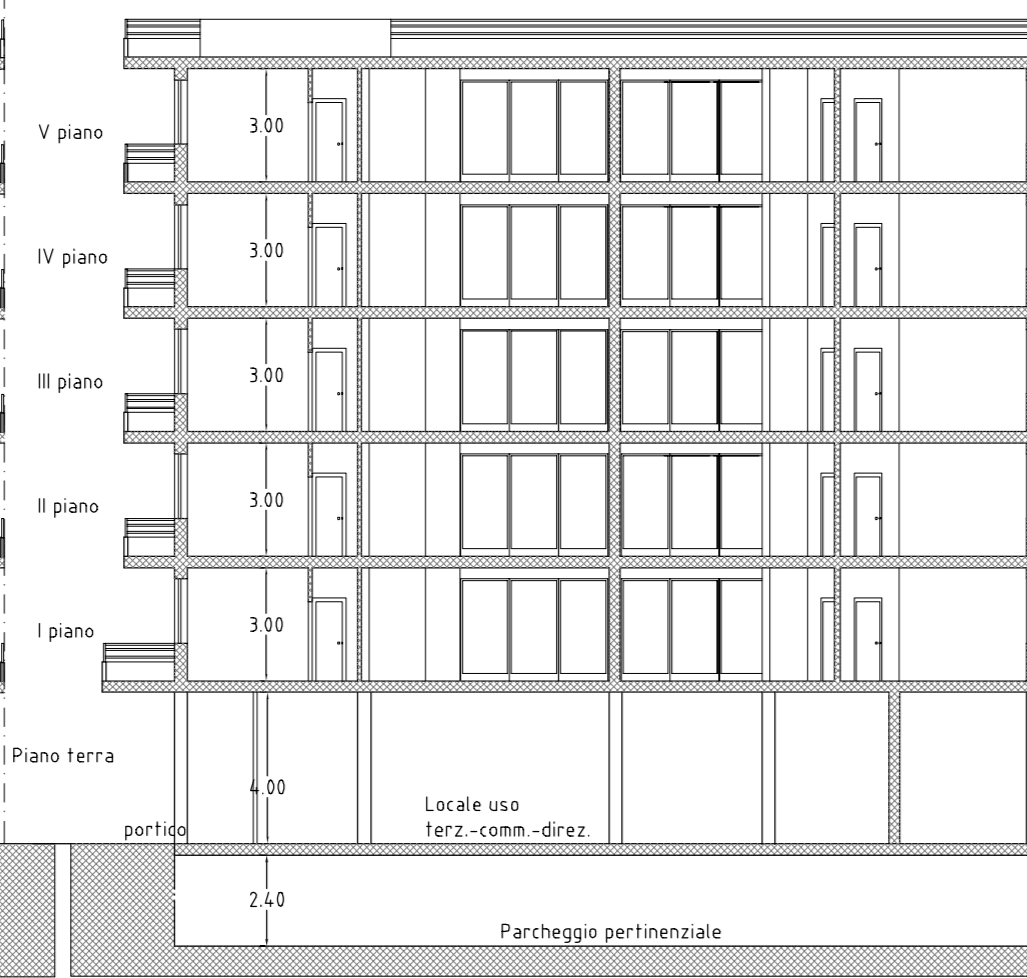
SEZIONE B-B
