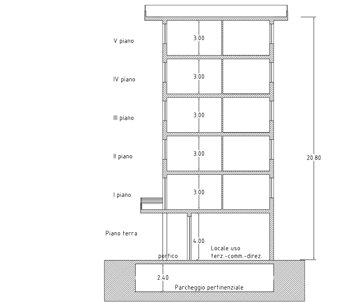
SEZIONE B2-B2
